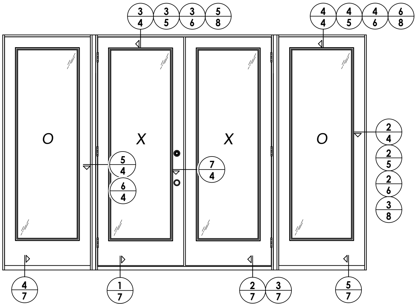
ELEVATION OXXO
